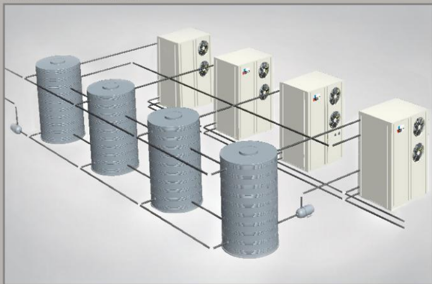
恒温型热泵热水机组系统图
